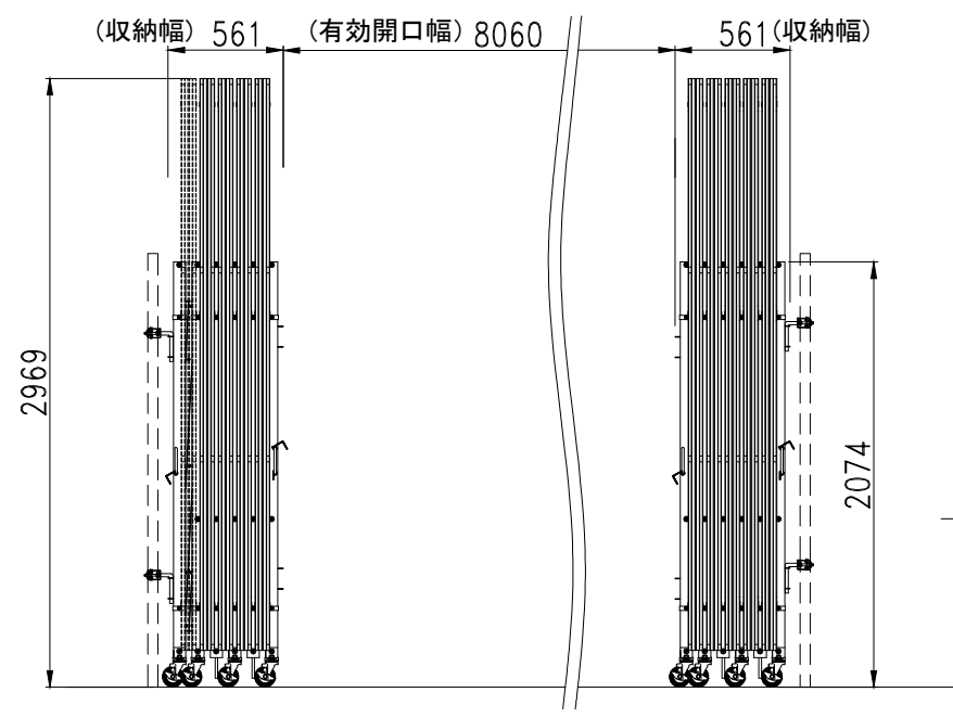
立面図 (収納時)
