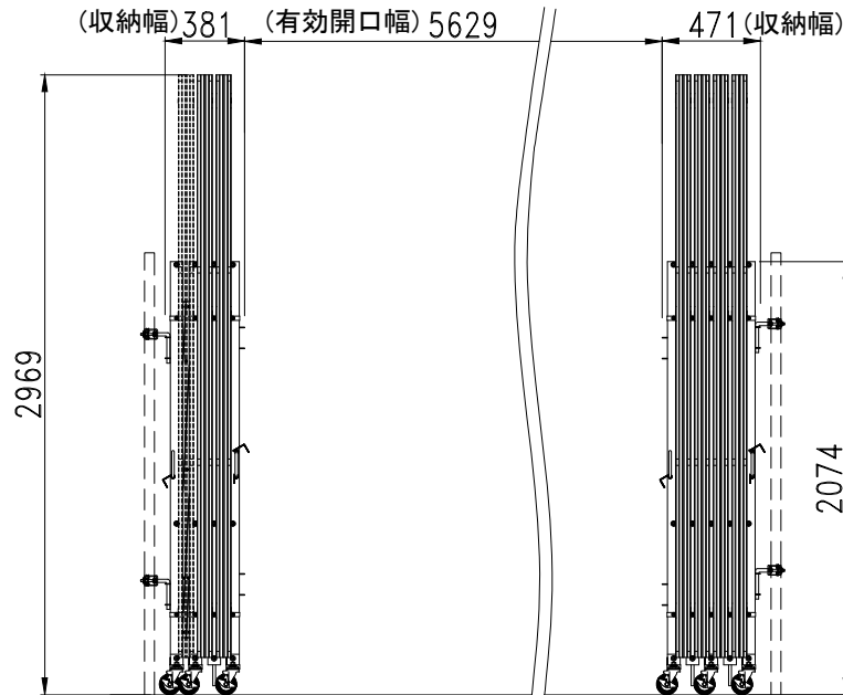
立面図 (収納時)
