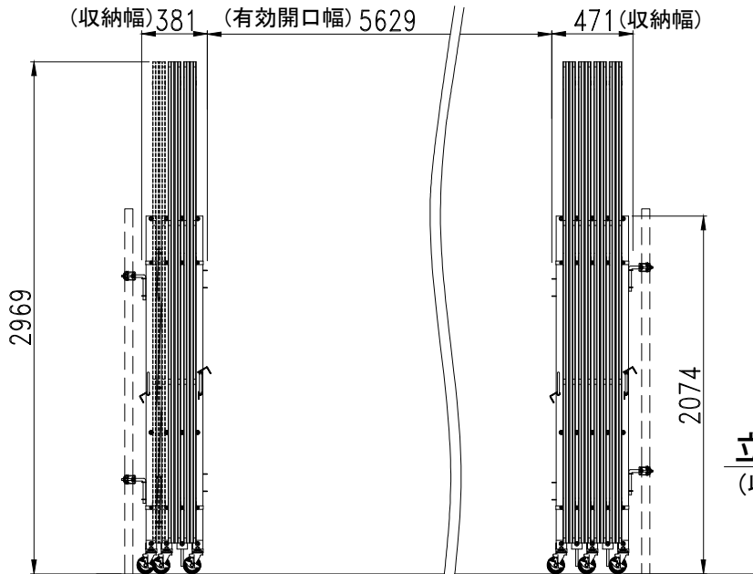
立面図
