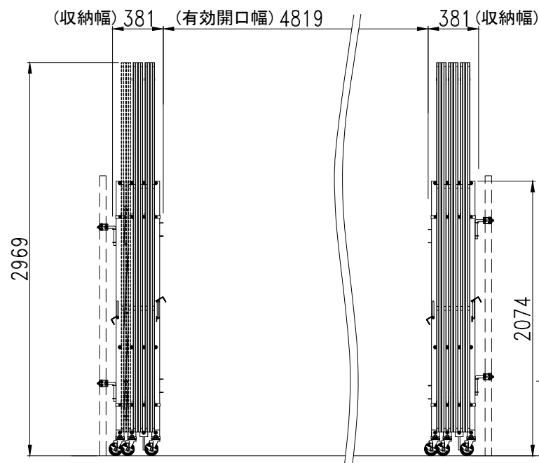
立面図 (収納時)
