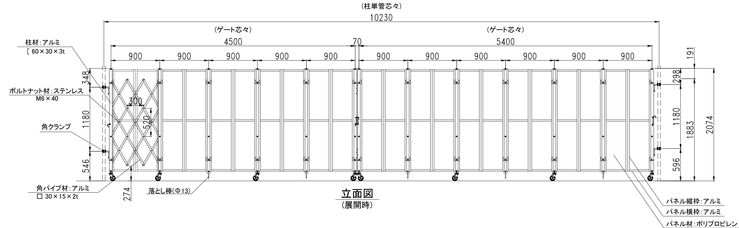
平面図 (展開時)
