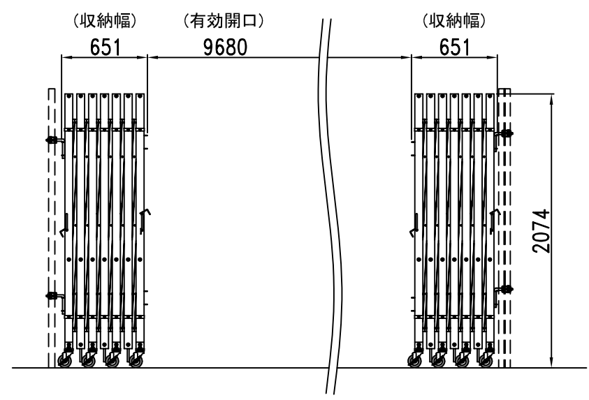
立面図 (収納時) S=1:30
