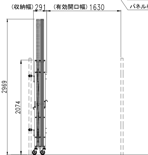
立面図 (収納時)
